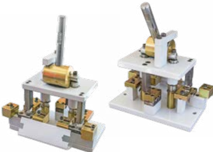
ESTAMPO PARA USINAGEM DA MÃO DE AMIGO
